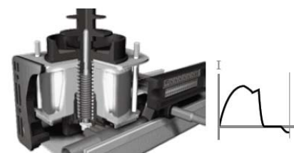
ISM v zapnutém stavu - magnetický akční člen vybuzený a připravený pro otevření
