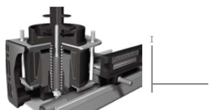
ISM ve vypnutém stavu
