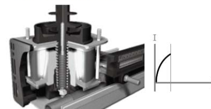
ISM ve vypnutém stavu - cívka magnetického pohonu začíná být buzena
